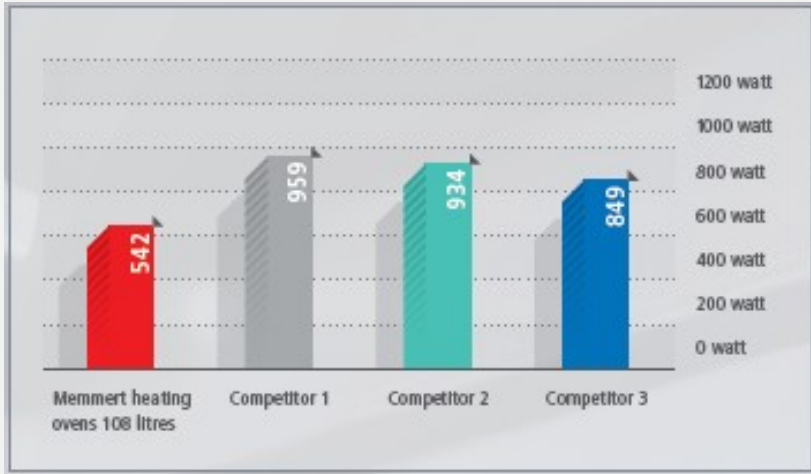
פליטת חום ב-250°C כאשר הקלפה להחלפת אויר סגורה
